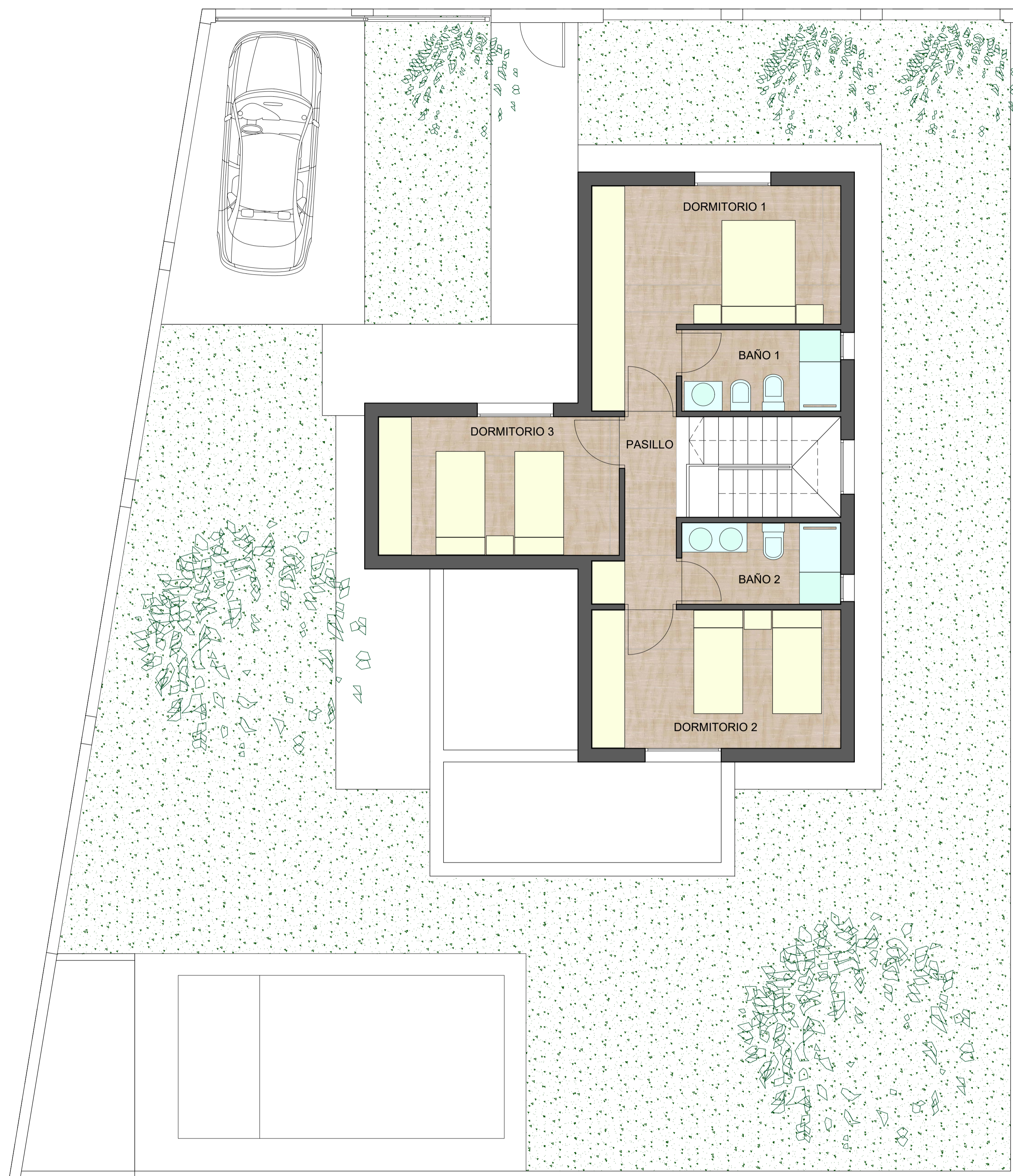
PLANTA BAJA
